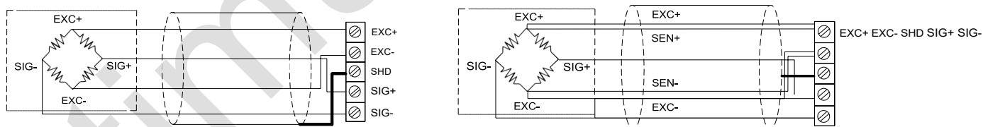
проводное подключение датчика
