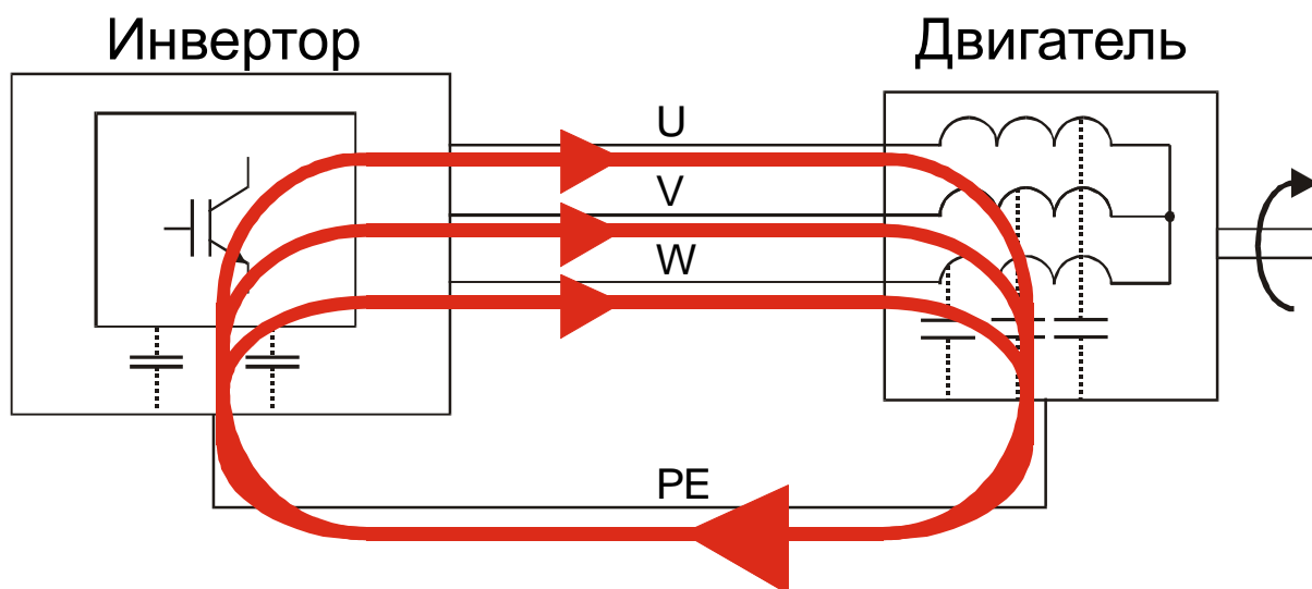
Рис. 1. Упрощенная схема протекания тока нулевой составляющей
