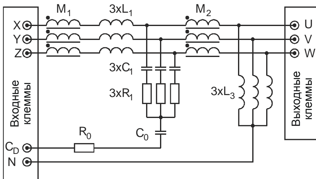
Рис. 2. Структура фильтра нулевой составляющей типа EFSZ
