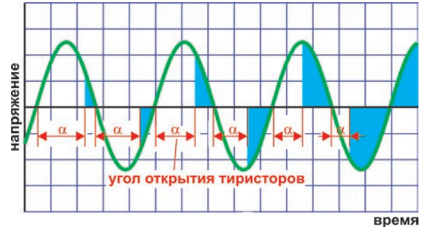
Формирование выходного напряжения УПП изменением угла открытия тиристоров
