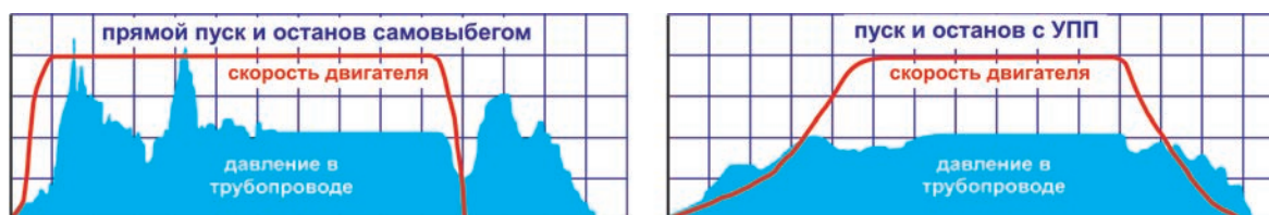
Устранение гидравлических ударов в трубопроводе
