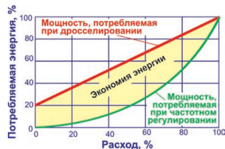
Экономия электроэнергии в насосном оборудовании
