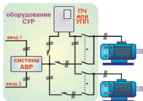
Пример станции управления типа СУР с возможностью каскадного включения двигателей
