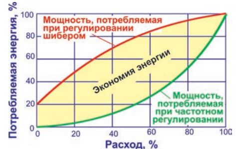
Экономия электроэнергии в вентиляторном оборудовании
