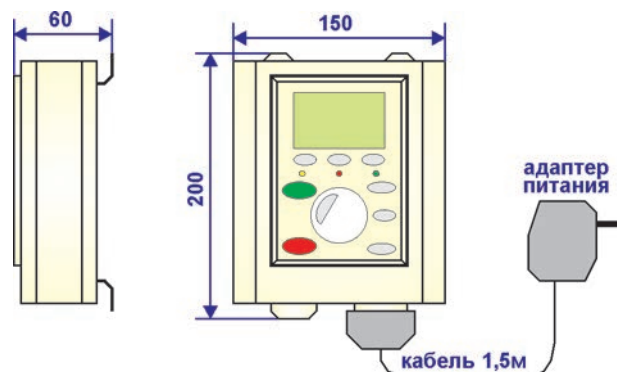
Габаритные размеры пульта дистанционного управления
