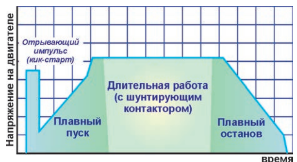
Типовая диаграмма напряжения на двигателе при работе УПП
