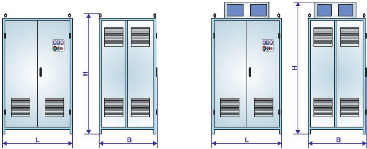
рисунок УППВ-1 (охлаждение воздушное естественное)
