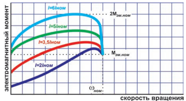
Механические характеристики двигателя при работе с УПП при различных значениях токоограничения в процессе пуска
